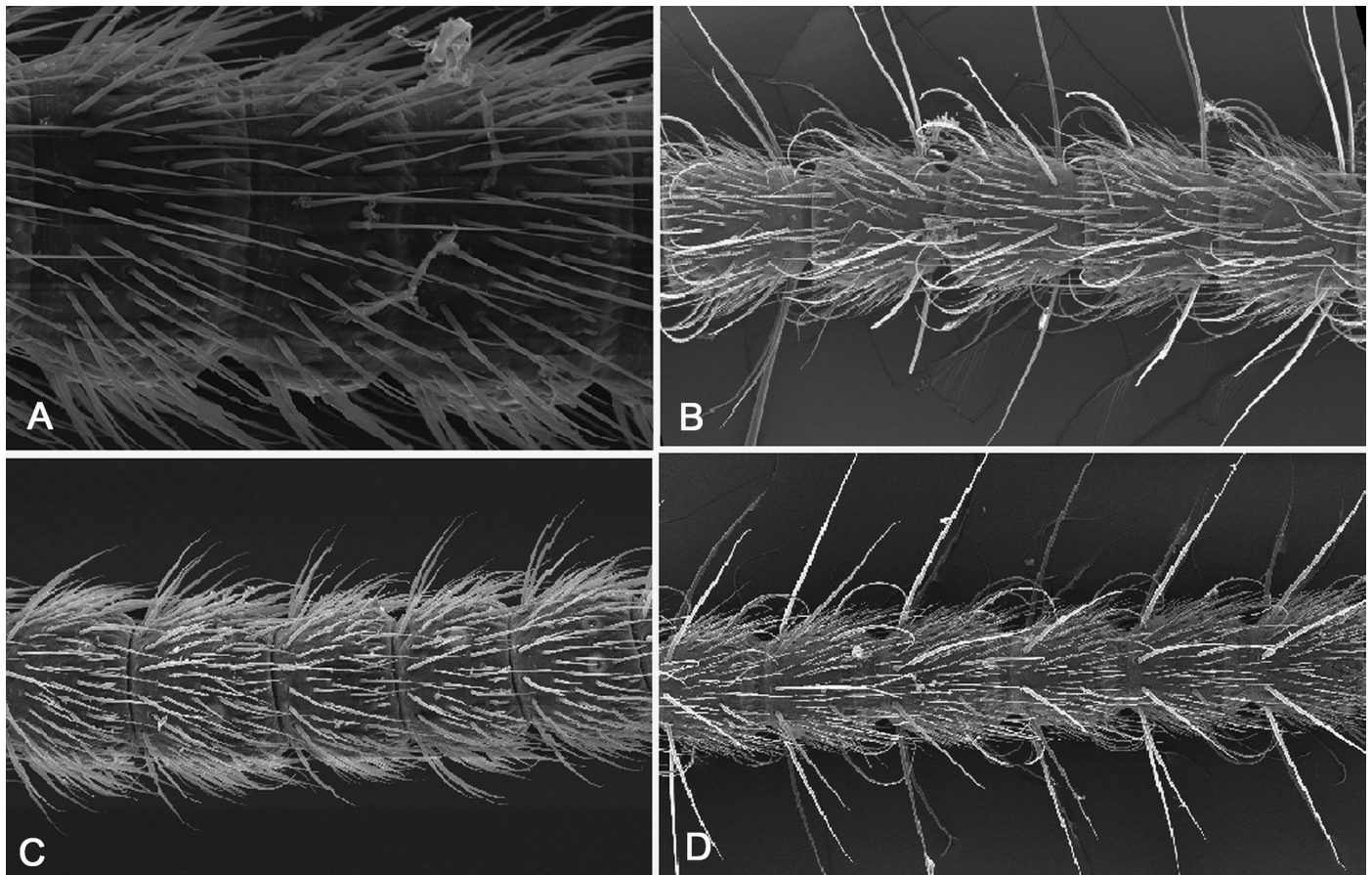
Fig. 1. SEM photos of the flagellum mid-section of N. hexadactyla (A), S. abbreviatus (B), S. vicinus (C) and S. borellii ( \times 140 ) (D).
